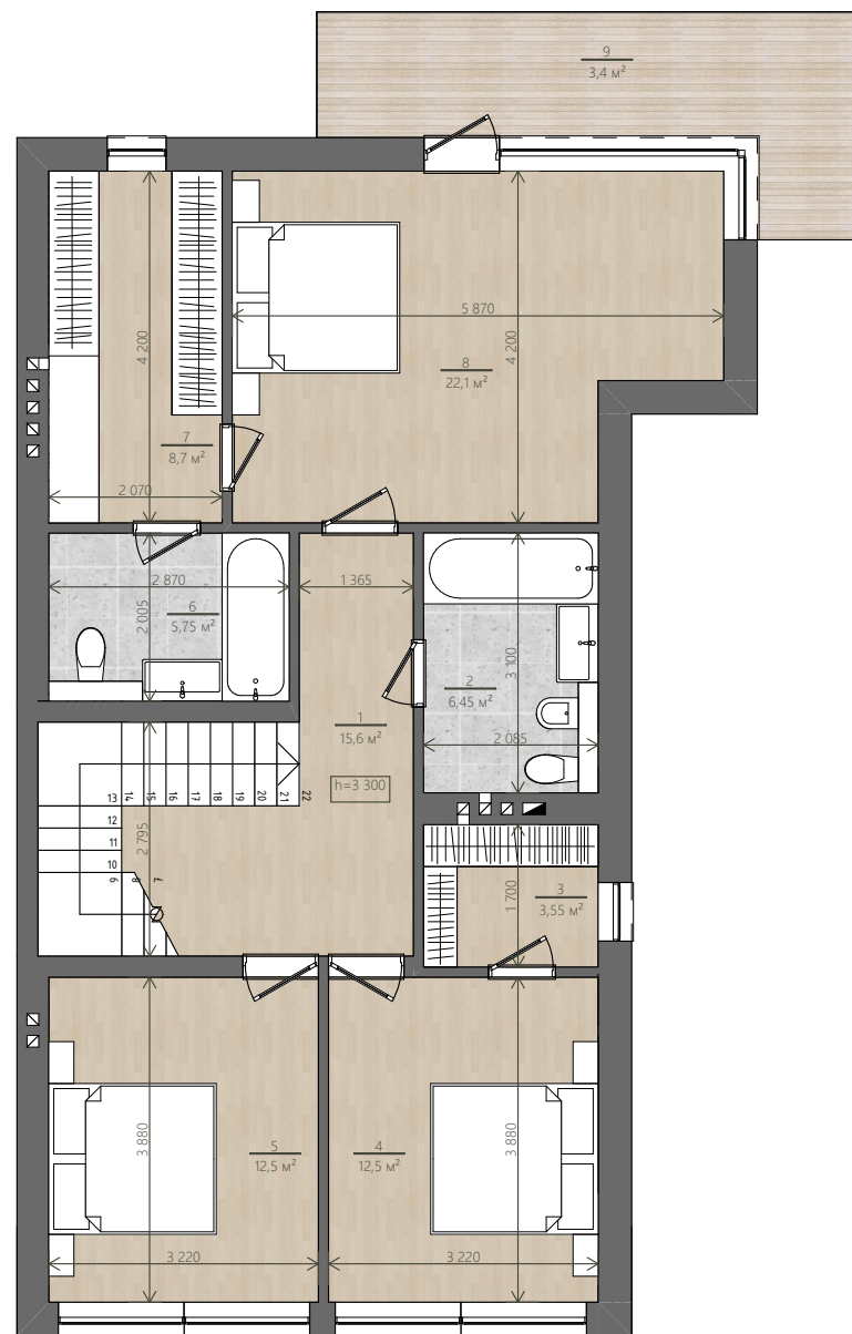
Другий поверх
