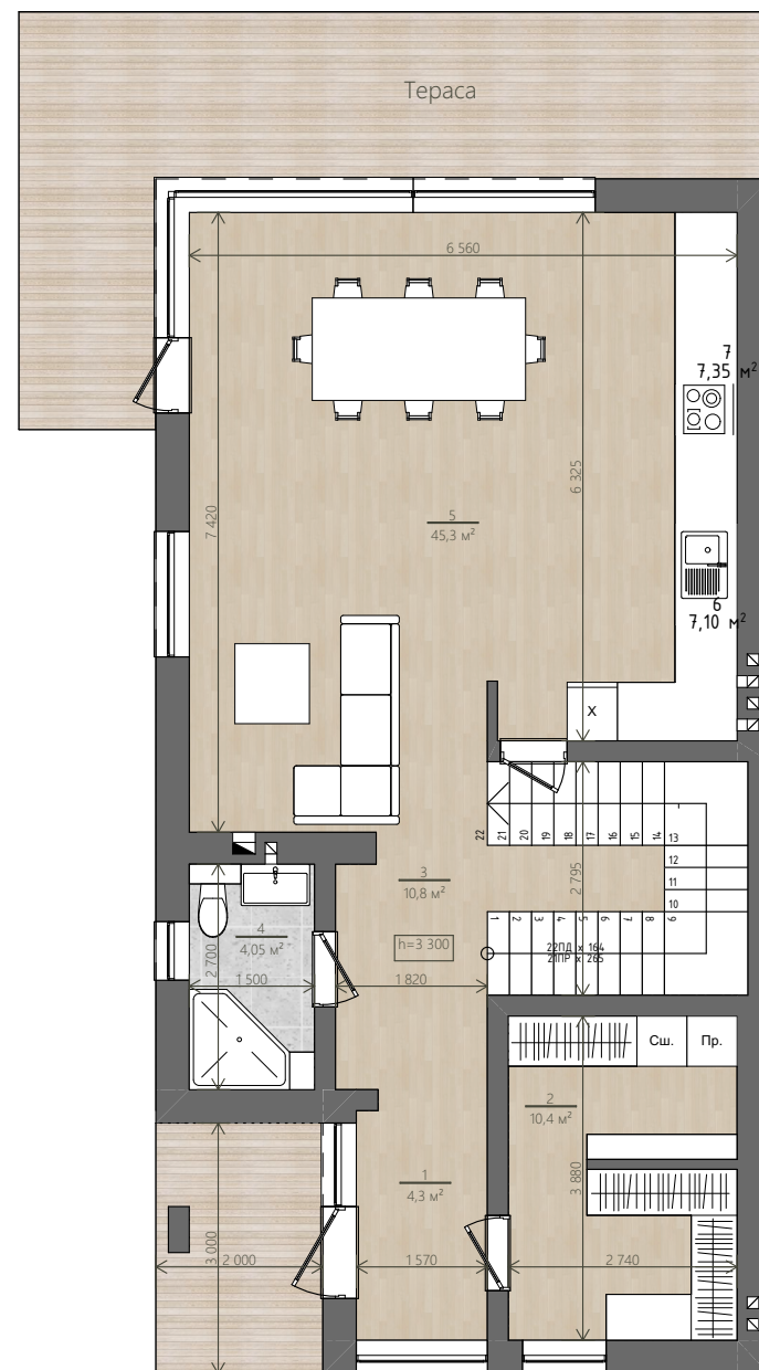
Перший поверх
