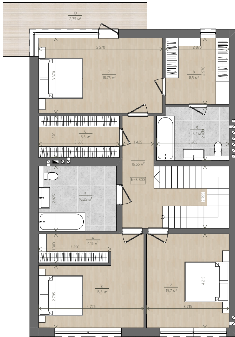
Другий поверх
