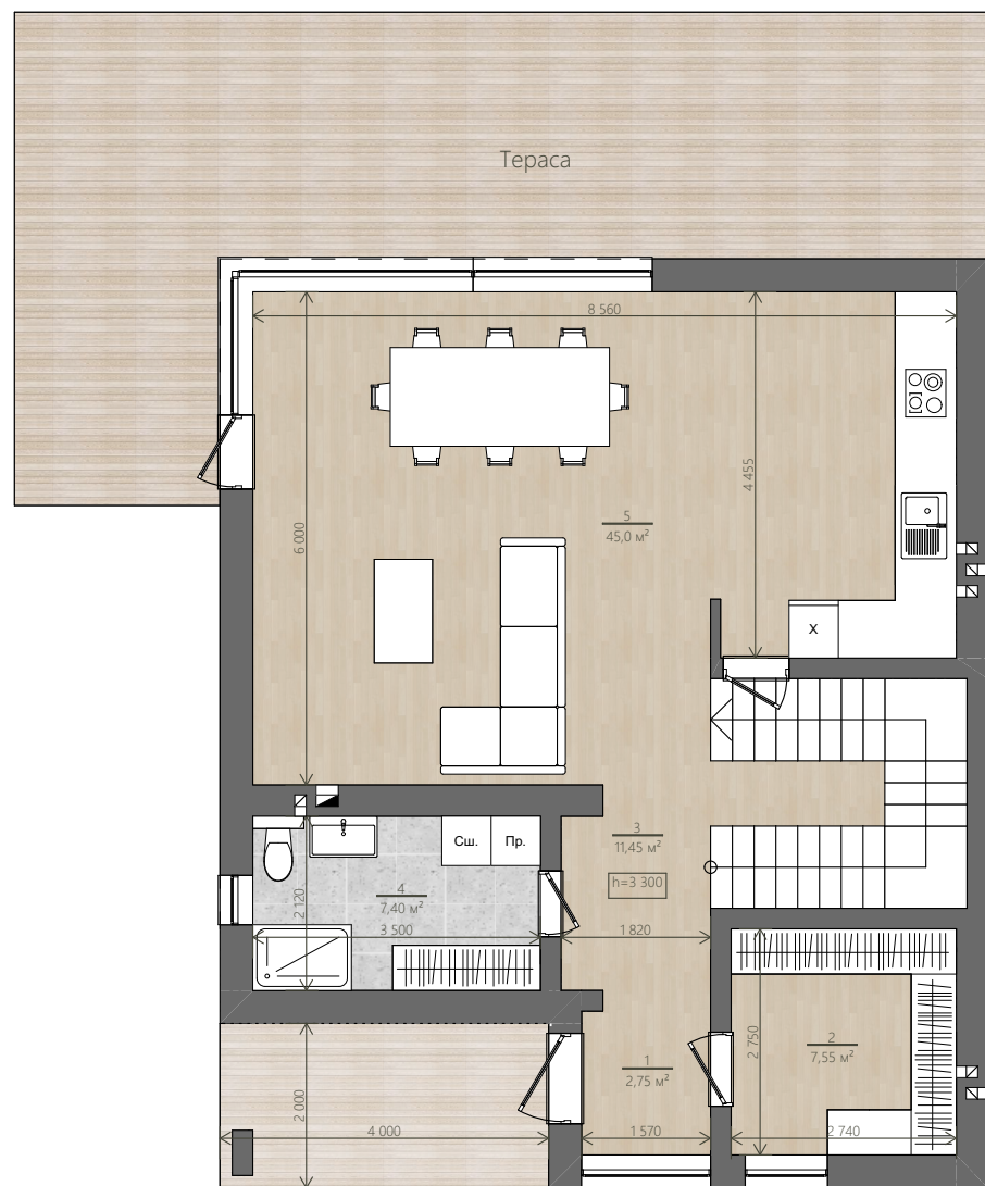
Перший поверх
